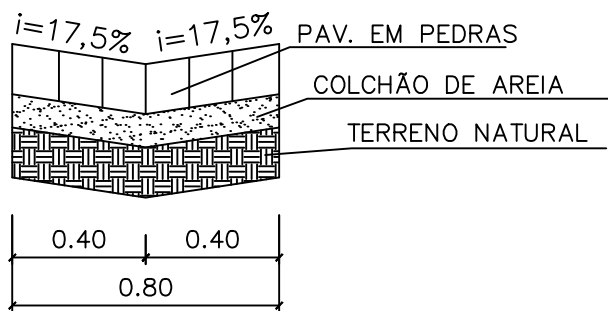
DETALHE DE SARJETA DUPLA (SEÇÃO)
