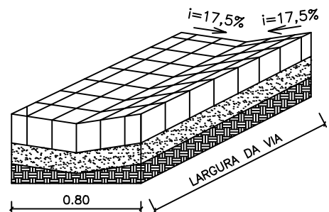
DETALHE DE SARJETA DUPLA (PERSPECTIVA)
